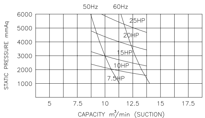
GTW-125A
